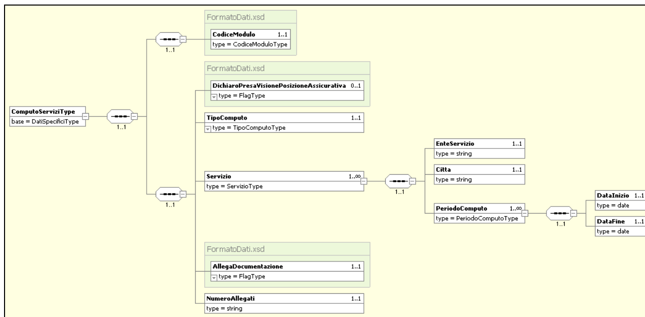
Figura 1 – CompuoServiziType
